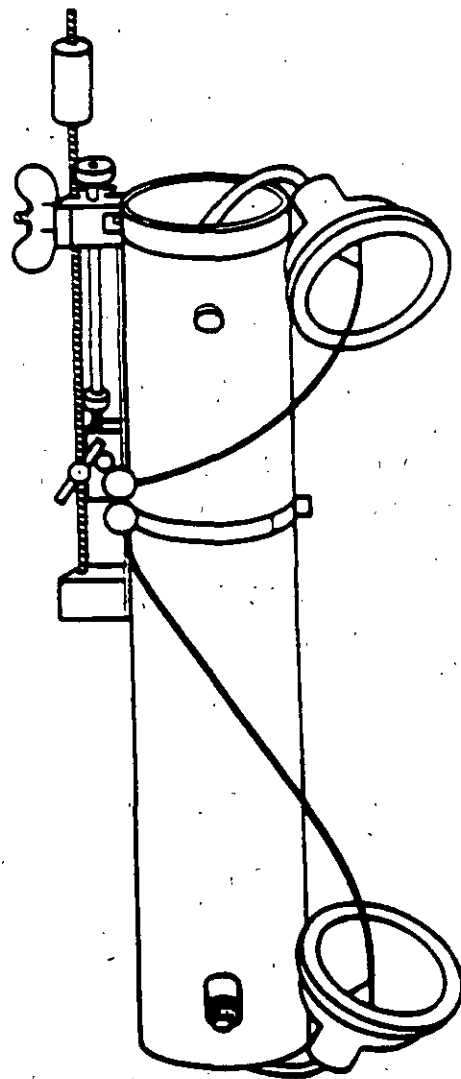
Van Dorn Sampler
